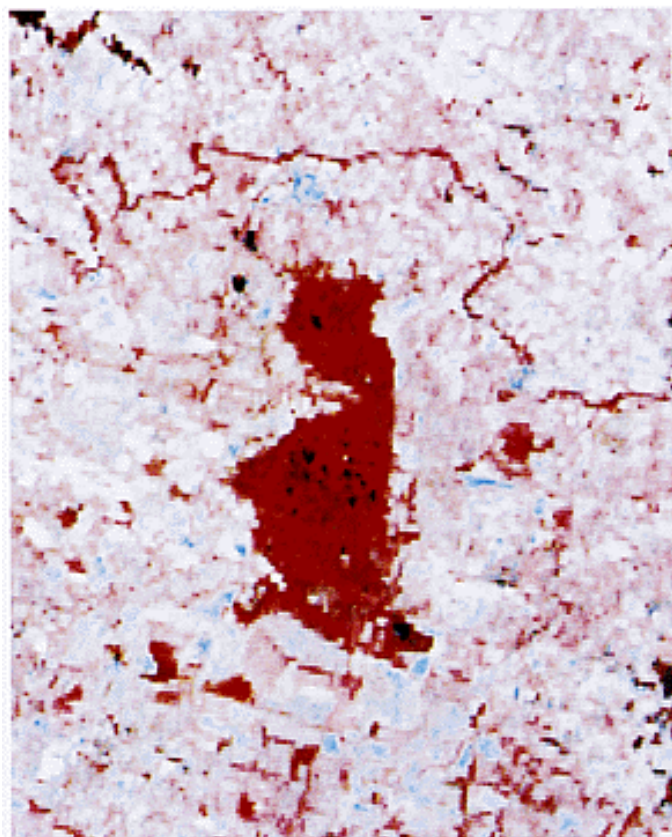
4.1.1. France/Area: Carcassonne Landsat TM 4.2.1. 1:100 000, July 1988
