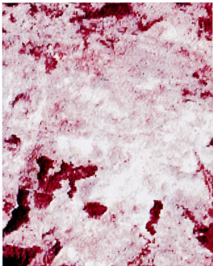
3.2.1. France/Area: causse de Sauveterre Landsat TM 4.2.1. 1:100 000, August 1989
